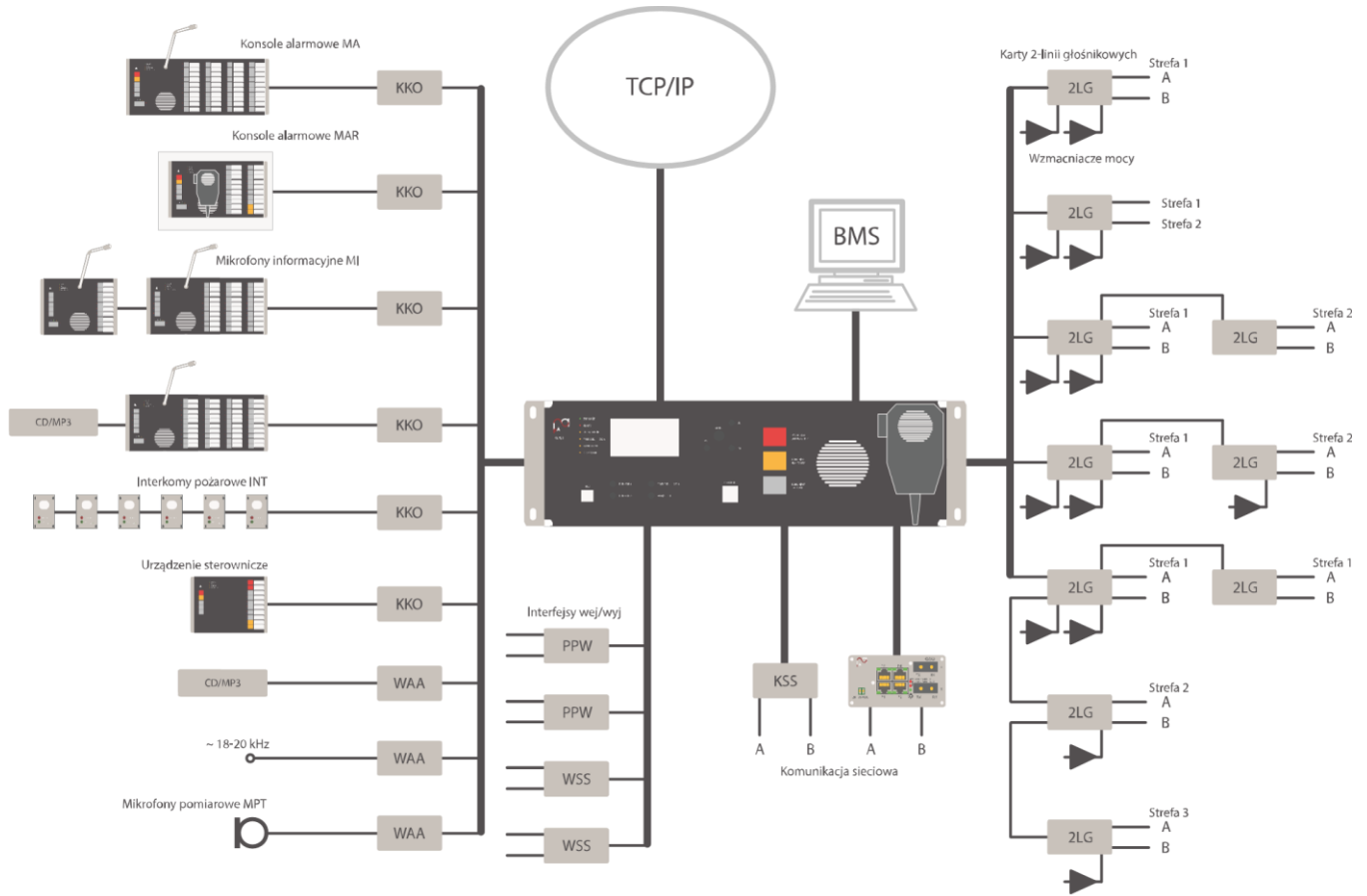
Konfiguracja podstawowa
